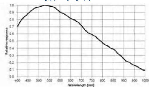
CK-U600MI-19RS 响应曲线
