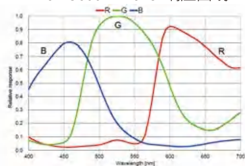
CK-U600CI-19RS 响应曲线
