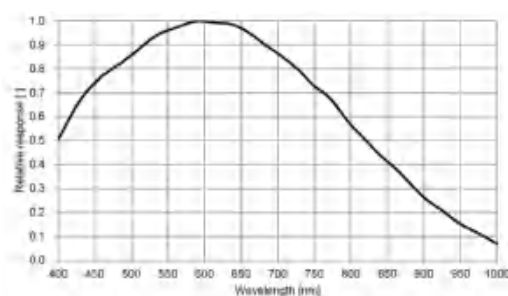
CK-S500MI-24GS 量子效率
