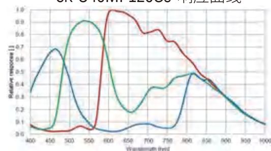
CK-U40CI-126GS 响应曲线
