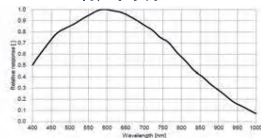
CK-U40MI-126GS 响应曲线
