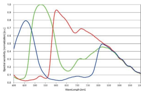
CK-U160CI-66GS 响应曲线
