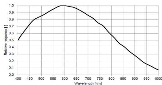
CK-U160MI-66GS 响应曲线
